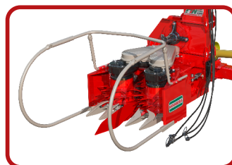
Tombador com regulagens que facilita a colheita em várias culturas
